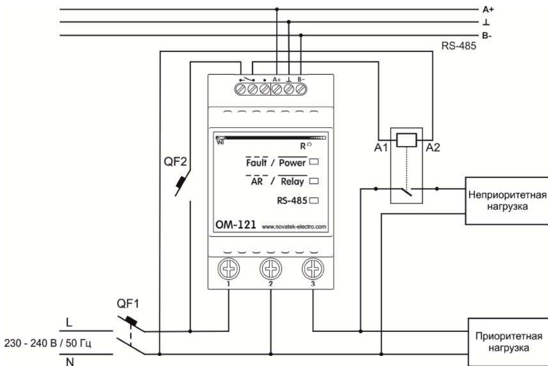
Рисунок 3 – Схема подключения в режиме ограничения мощности
